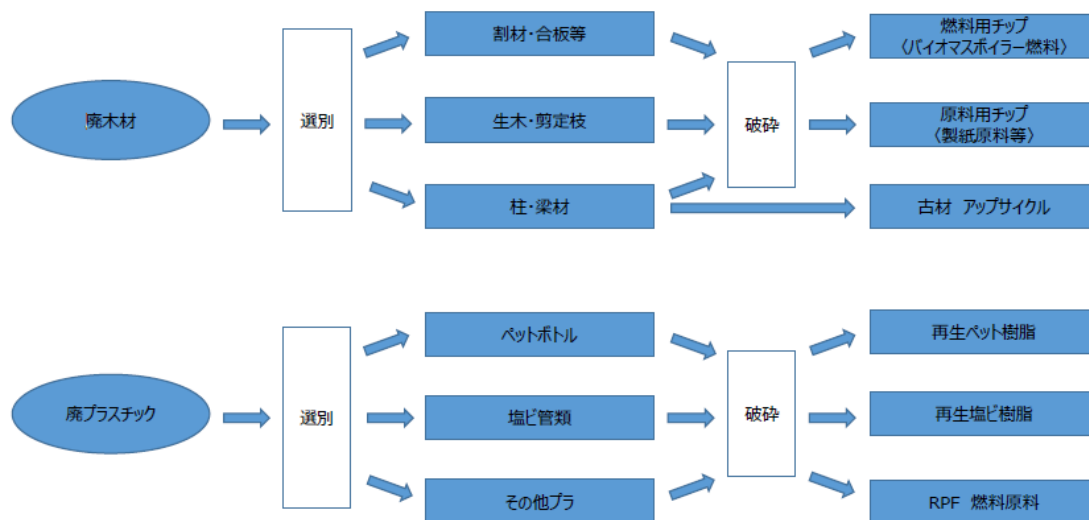
産業廃棄物処理フロー
